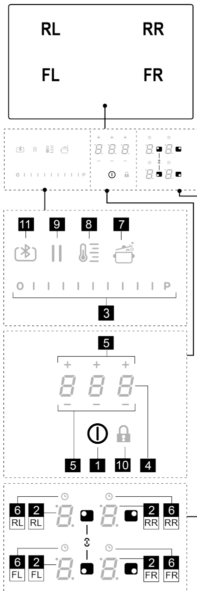
Pannello di controllo mod.804P
