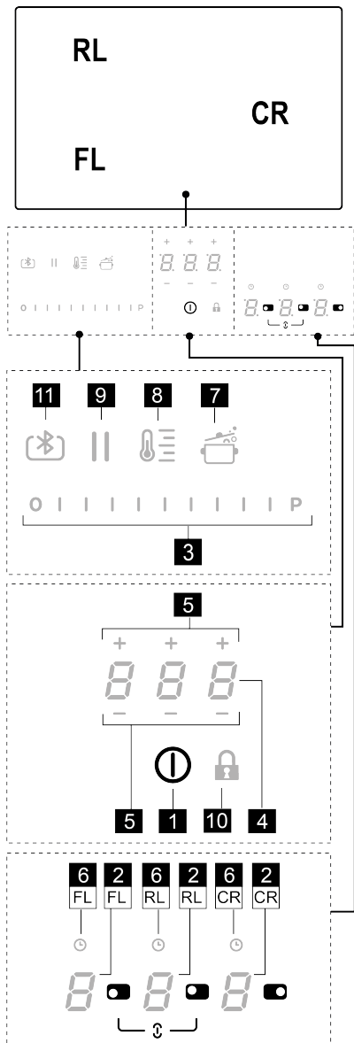
Mudeli 803P juhtpaneel
